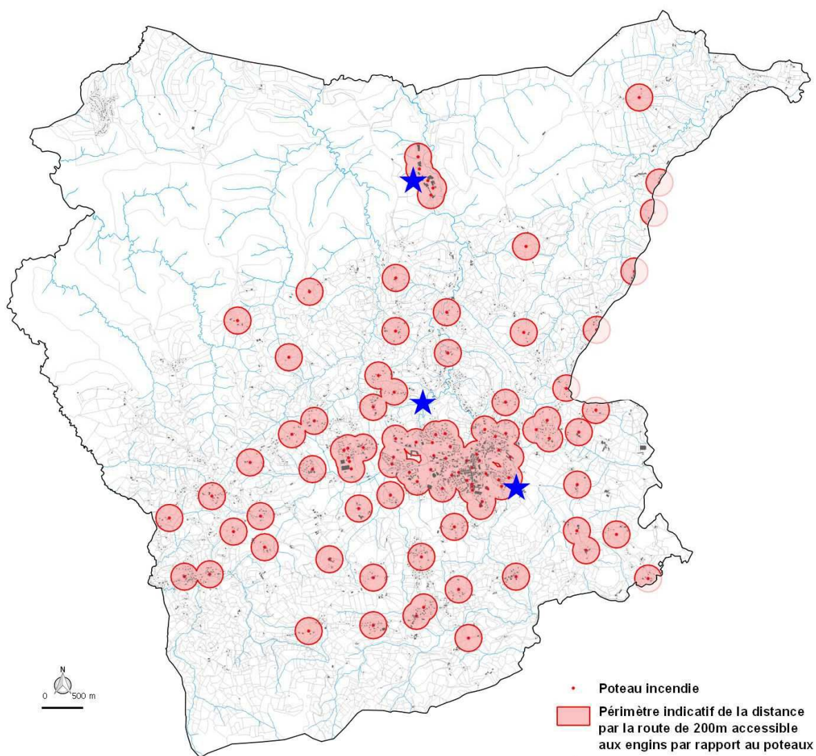
Schématisation de la couverture incendie
